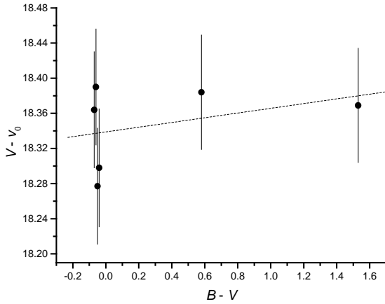
Figura 5. Ajuste lineal (V - v_0) vs. (B - V) para la obtención de \epsilon y \zeta_v . Los valores calculados son \epsilon = 0.0268 \pm 0.0337 y \zeta_v = 18.3388 \pm 0.0229 .
