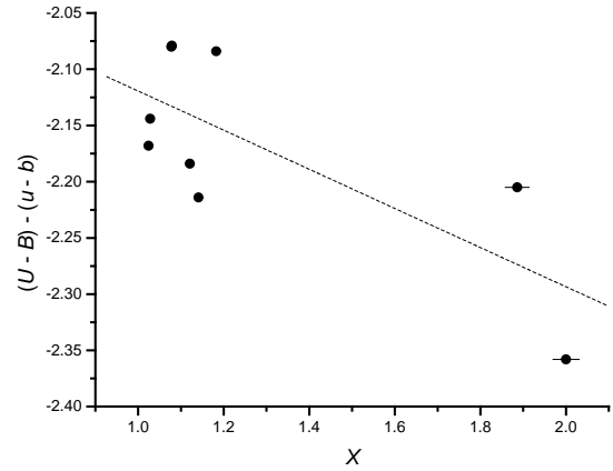
Figura 4. Ajuste lineal (U - B) - (u - b) vs. X para la obtención de K'_{ub} . El valor calculado es K'_{ub} = 0.1742 \pm 0.0593 .
