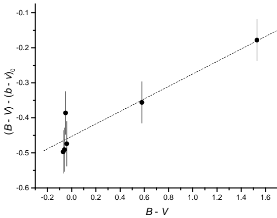
Figura 6. Ajuste lineal (B - V) - (b - v)_0 vs. (B - V) para la obtención de \mu y \zeta_{bv} . Los valores calculados son \mu = 1.2169 \pm 0.0440 y \zeta_{bv} = -0.5510 \pm 0.0320 .
