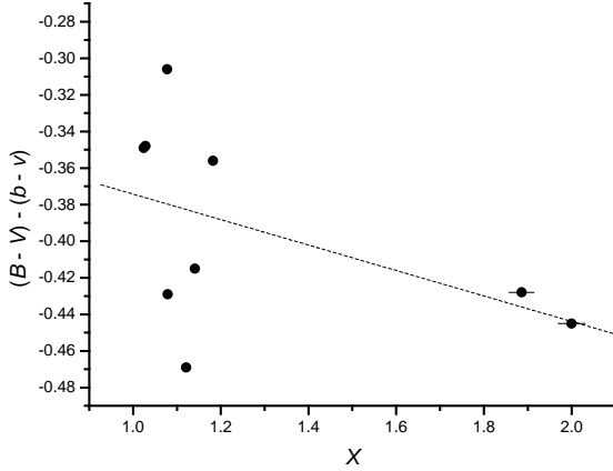
Figura 3. Ajuste lineal (B - V) - (b - v) vs. X para la obtención de K'_{bv} . El valor calculado es K'_{bv} = 0.0696 \pm 0.0484 .
