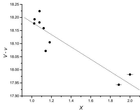
Figura 2. Ajuste lineal ( V-v ) vs. X para la obtención de K'_v . El valor calculado es K'_v = 0.2356 \pm 0.0410 .
