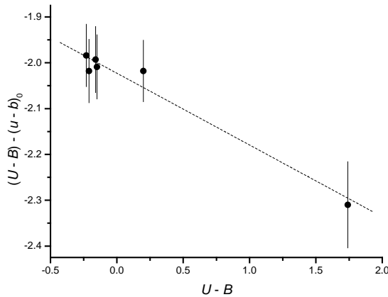
Figura 7. Ajuste lineal (U - B) - (u - b)_0 vs. (U - B) para la obtención de \psi y \zeta_{ub} . Los valores calculados son \psi = 0.8645 \pm 0.0137 y \zeta_{ub} = -1.7487 \pm 0.0292 .
